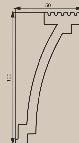
SCHITA TEHNICA
